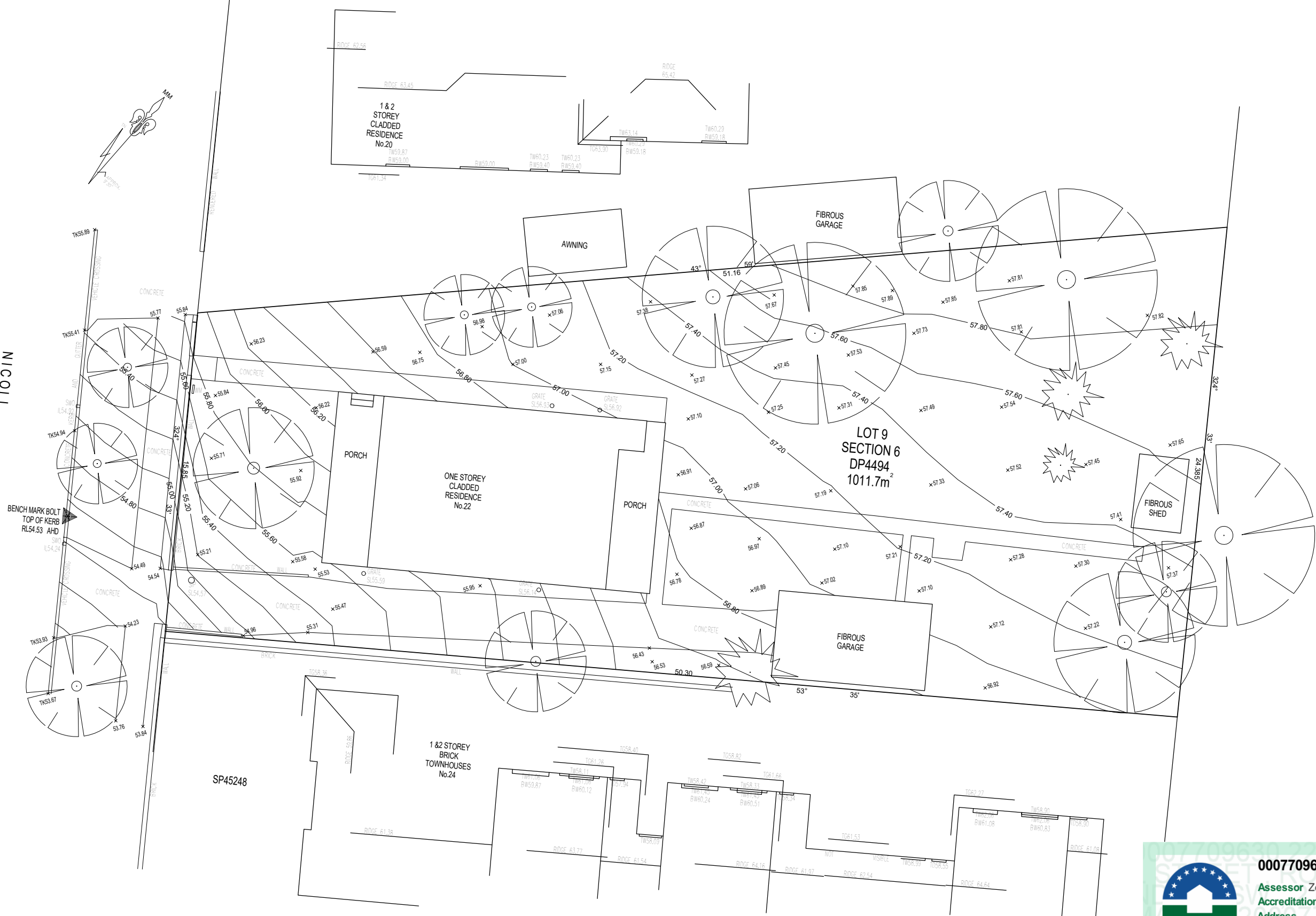
1 SITE SURVEY 1 : 200
